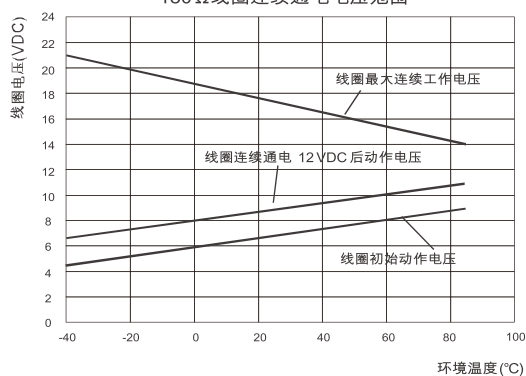
180Ω线圈连续通电电压范围
