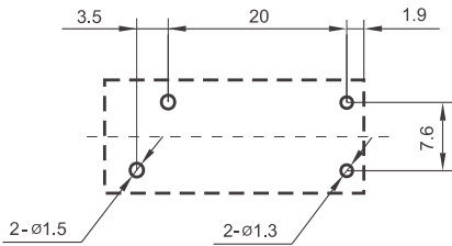
安装孔尺寸 PCB LAYOUT (底视图 Bottom View)
